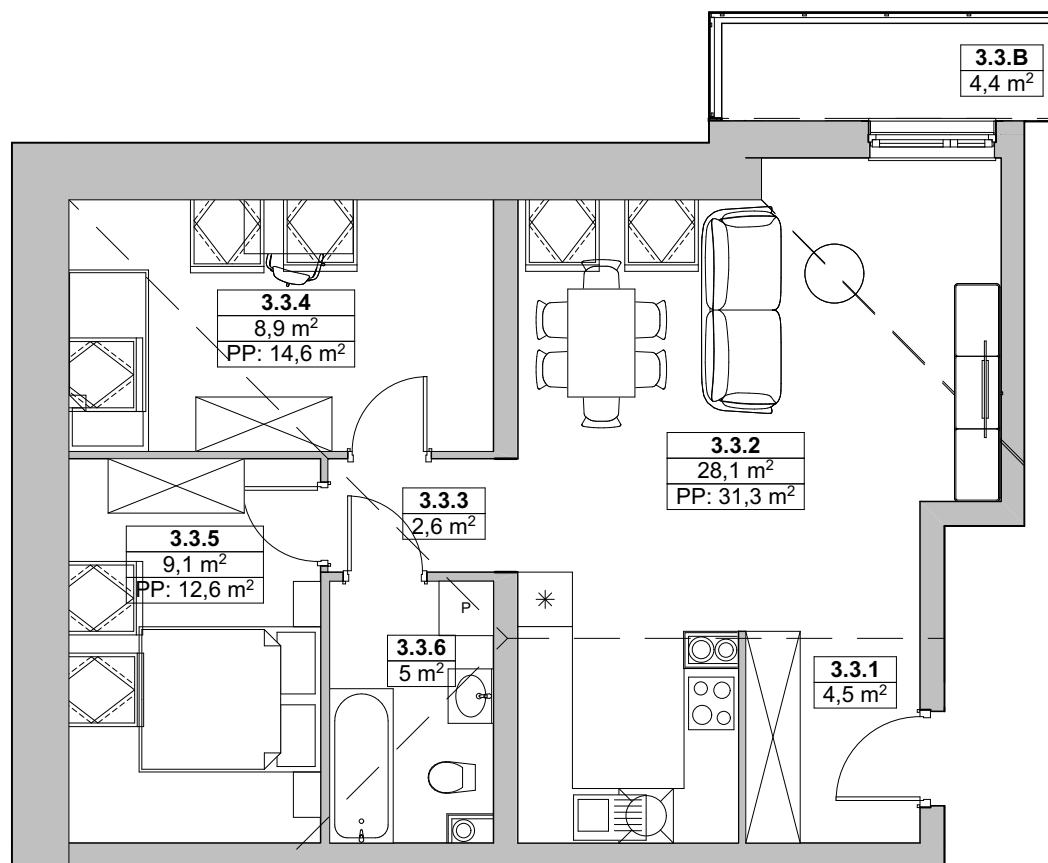
ZESTAWIENIE POWIERZCHNI pom.pom. = pomieszczenie pomocnicze
