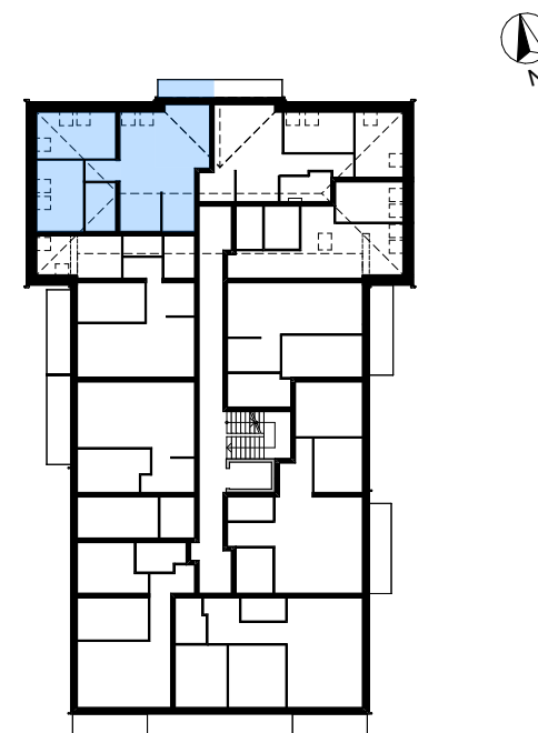
UKŁAD KONDYGNACJI 1:500
